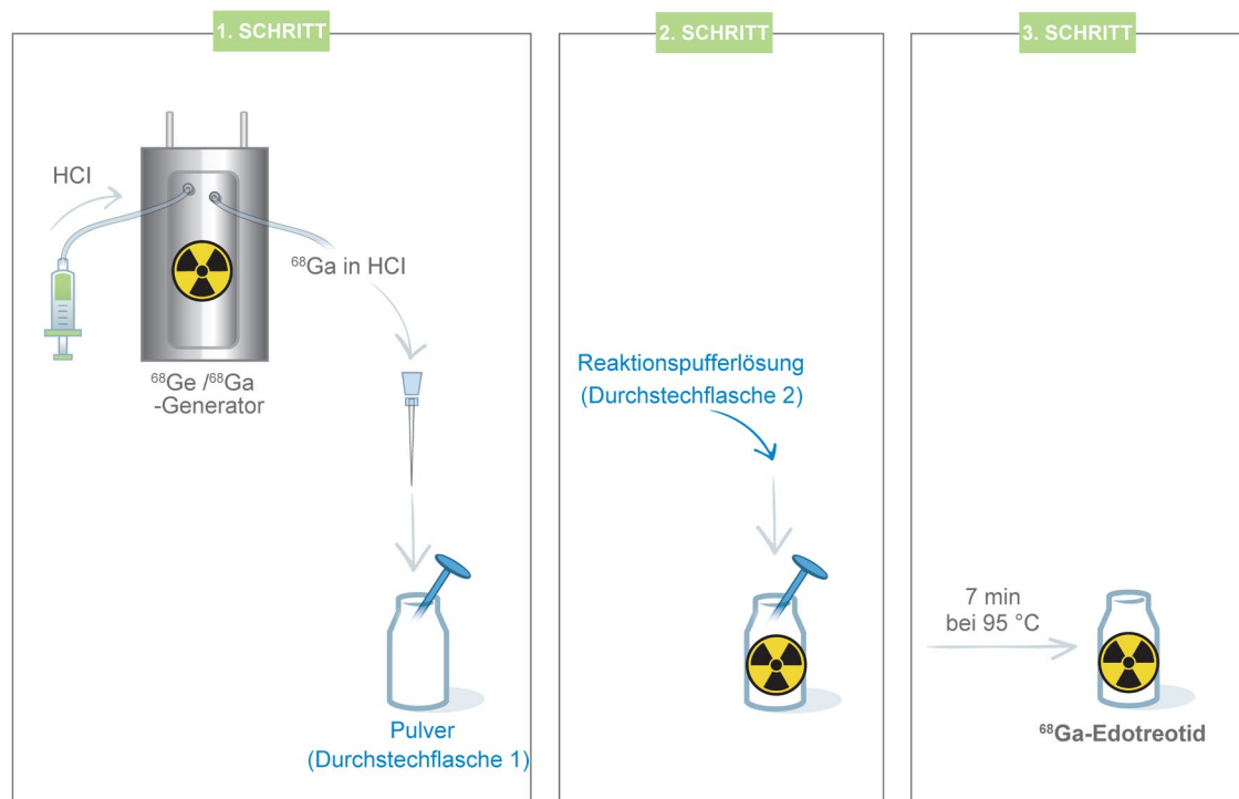
Abbildung 1 Verfahren zur radioaktiven Markierung mit dem GalliaPharm-Generator
